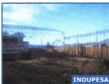
Fotos Nº 23 y 24 - Primera etapa de la construcción del muelle de descarga y cámara frigorífica.
